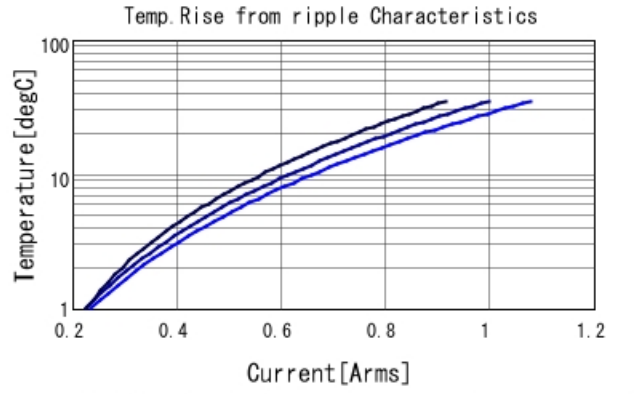
GRM1555C1H240JA01 Temp. rise — 500MHz — 700I
