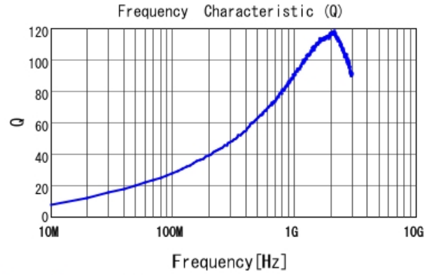
LQW18AN12NJ00 Q
