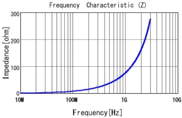
LQW18AN12NJ00 |Z|
