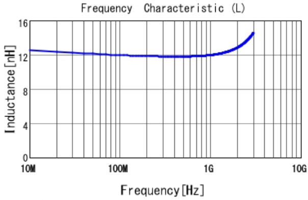
LQW18AN12NJ00 L
