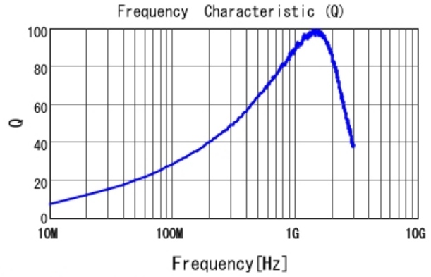
LQW18AN24NG00 Q
