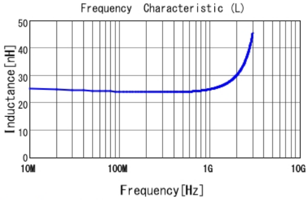
LQW18AN24NG00 L
