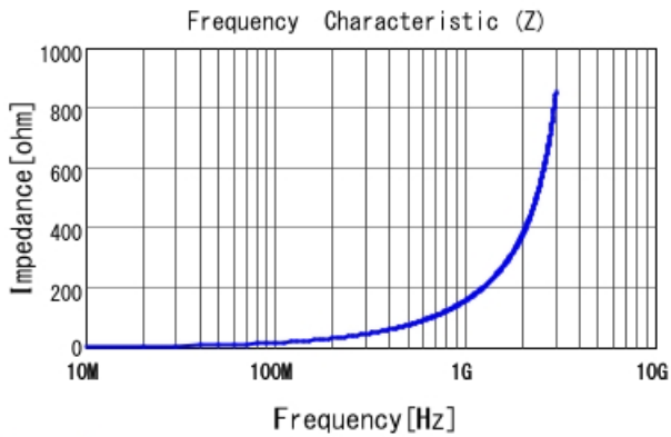
LQW18AN24NG00 |Z|
