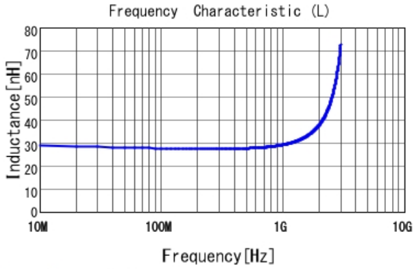
LQW18AN27NJ00 L
