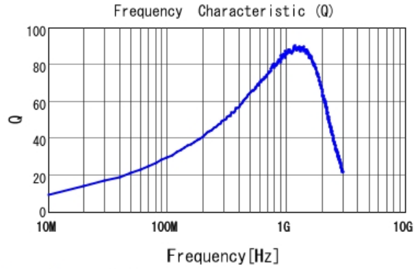
LQW18AN27NJ00 Q
