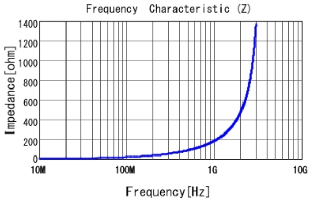
LQW18AN27NJ00 |Z|
