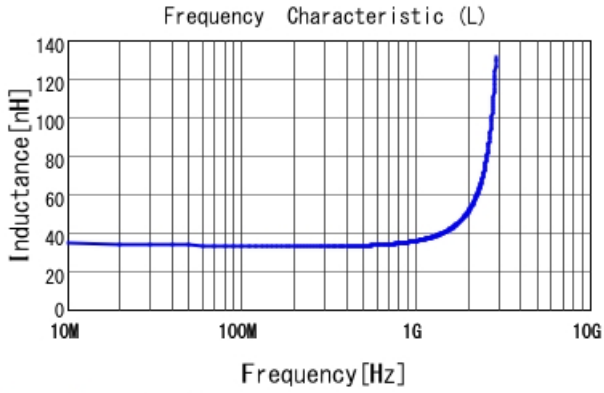
LQW18AN33NG00 L
