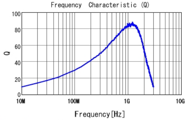
LQW18AN33NG00 Q
