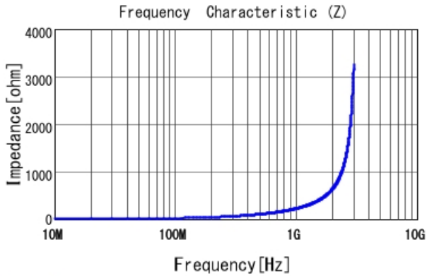
LQW18AN33NG00 |Z|
