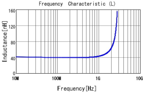
LQW18AN39NJ00 L
