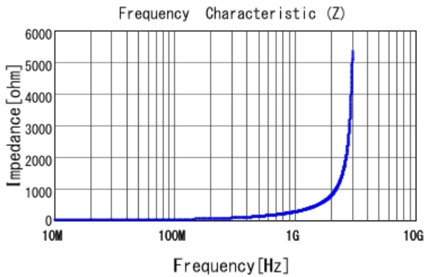
LQW18AN39NJ00 |Z|
