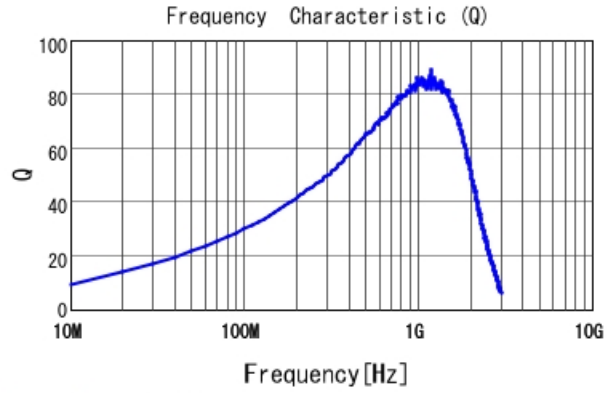
LQW18AN39NJ00 Q
