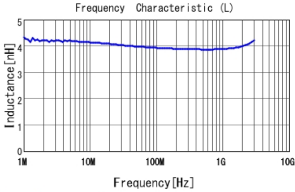
LQW18AN3N9B8Z L
