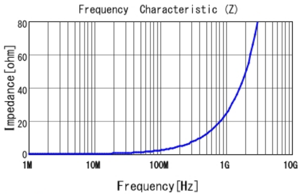
LQW18AN3N9B8Z |Z|
