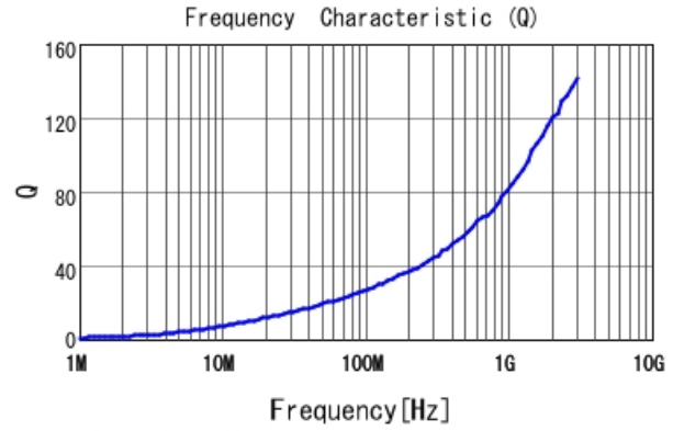
LQW18AN3N9B8Z Q
