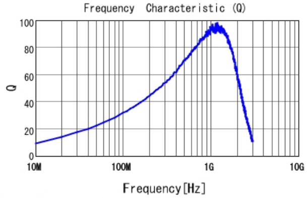
LQW18AN43NG00 Q
