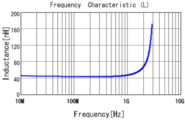
LQW18AN43NG00 L
