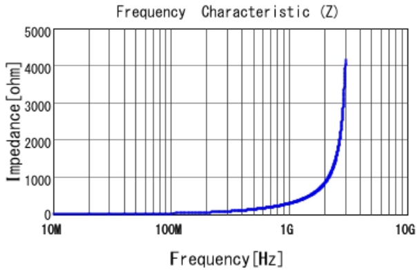
LQW18AN43NG00 |Z|
