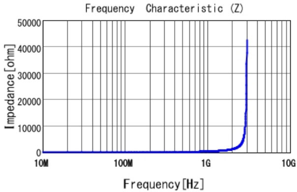
LQW18AN56NG00 |Z|
