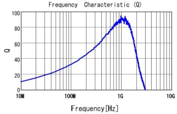
LQW18AN56NG00 Q
