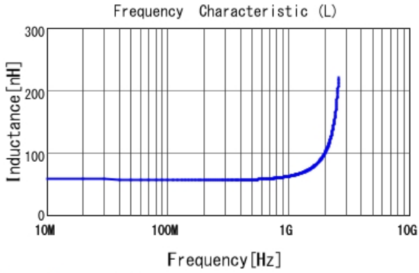
LQW18AN56NG00 L
