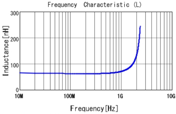
LQW18AN62NG00 L
