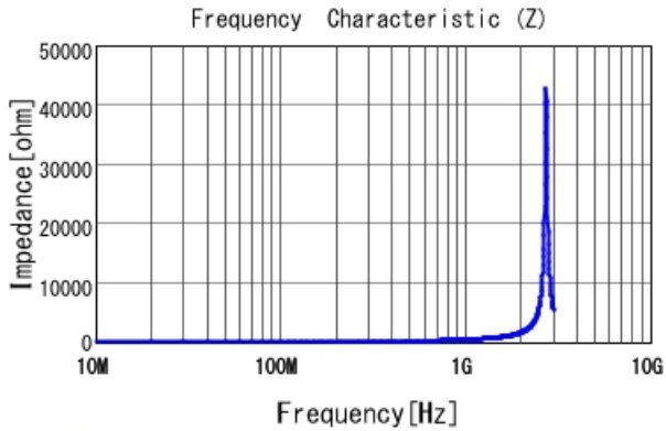
LQW18AN62NG00 |Z|
