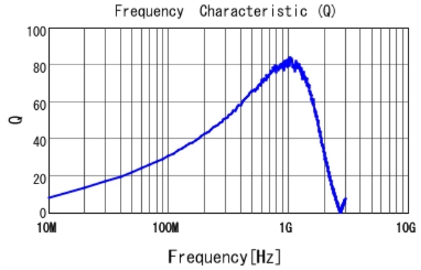
LQW18AN62NG00 Q
