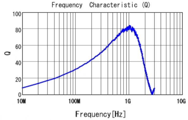
LQW18AN62NJ00 Q
