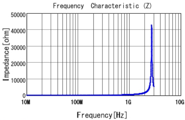
LQW18AN62NJ00 |Z|
