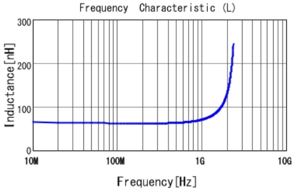
LQW18AN62NJ00 L
