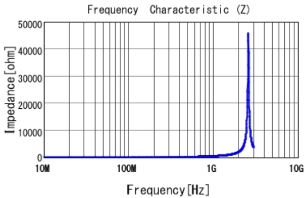
LQW18AN68NJ00 |Z|
