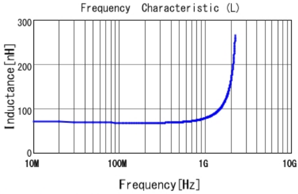
LQW18AN68NJ00 L
