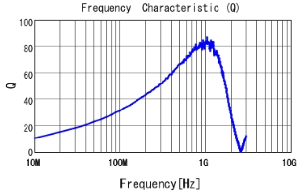
LQW18AN68NJ00 Q
