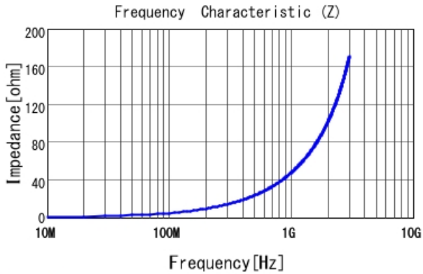
LQW18AN7N5C00 |Z|
