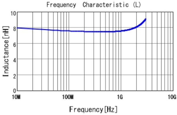
LQW18AN7N5C00 L
