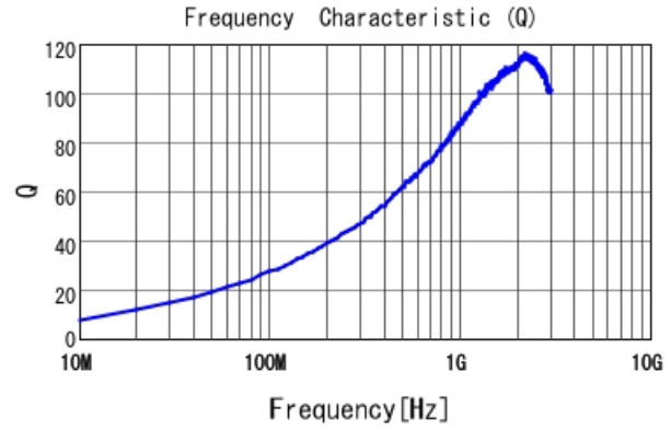
LQW18AN7N5C00 Q
