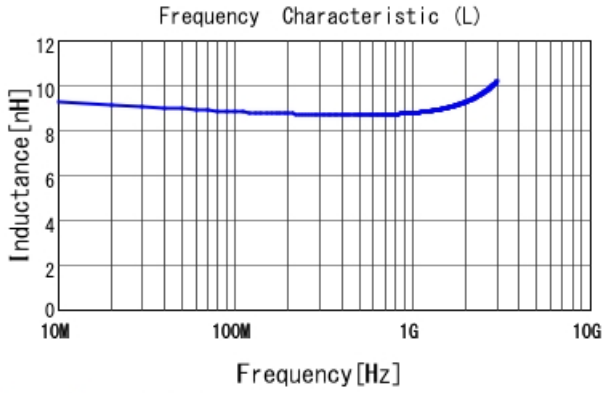
LQW18AN8N7D00 L
