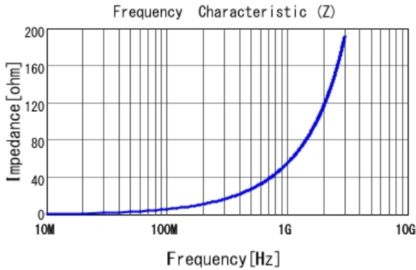
LQW18AN8N7D00 |Z|
