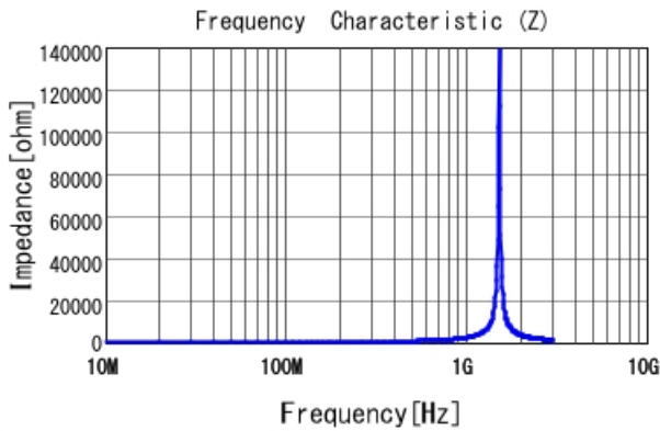
LQW18ANR22J00 |Z|
