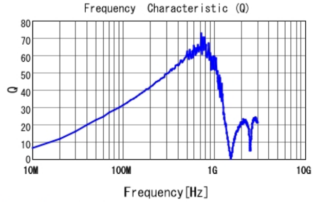
LQW18ANR22J00 Q
