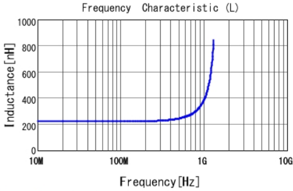
LQW18ANR22J00 L
