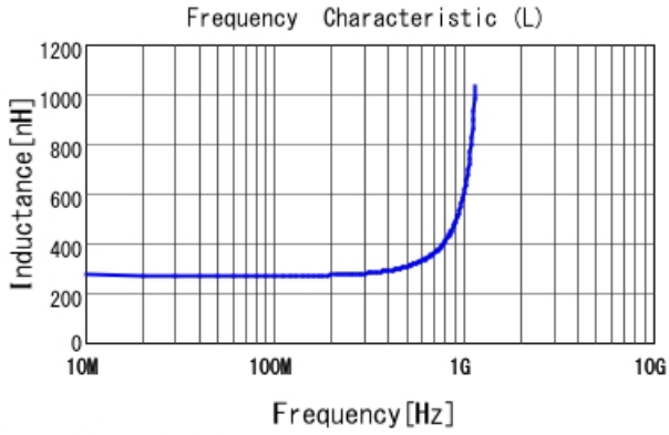
LQW18ANR27G00 L
