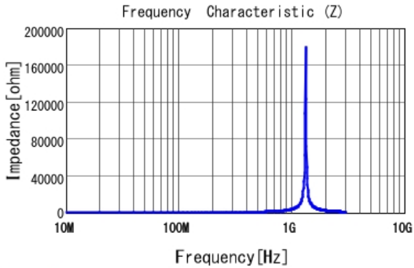
LQW18ANR27G00 |Z|
