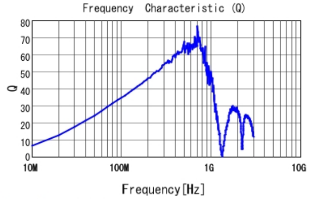
LQW18ANR27G00 Q
