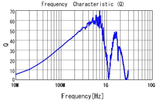
LQW18ANR39G00 Q
