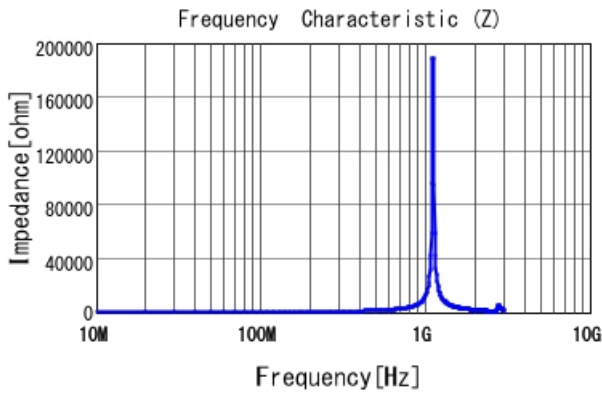
LQW18ANR39G00 |Z|
