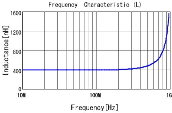
LQW18ANR39G00 L
