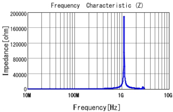
LQW18ANR39J00 |Z|
