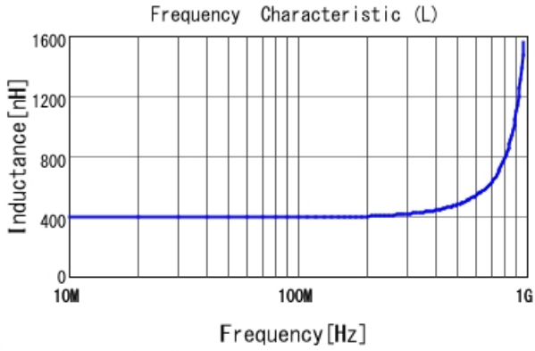
LQW18ANR39J00 L
