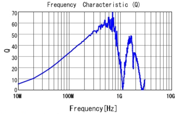
LQW18ANR39J00 Q
